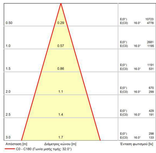
Κωνικό διάγραμμα για Έξοδοι φωτός 1 και 2
