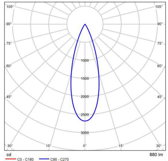
Πολικό διάγραμμα κατανομής φωτός για Έξοδοι φωτός 1 και 2
